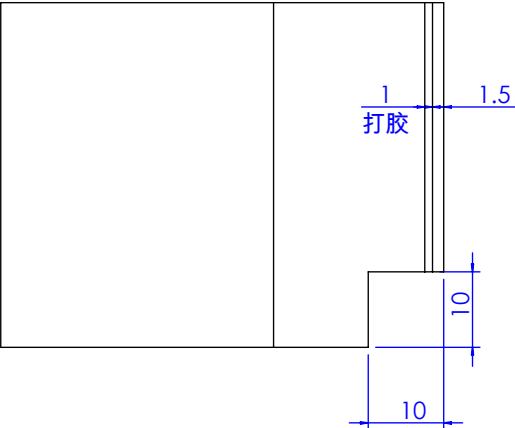
局部视图 AM 比例 1 : 1
