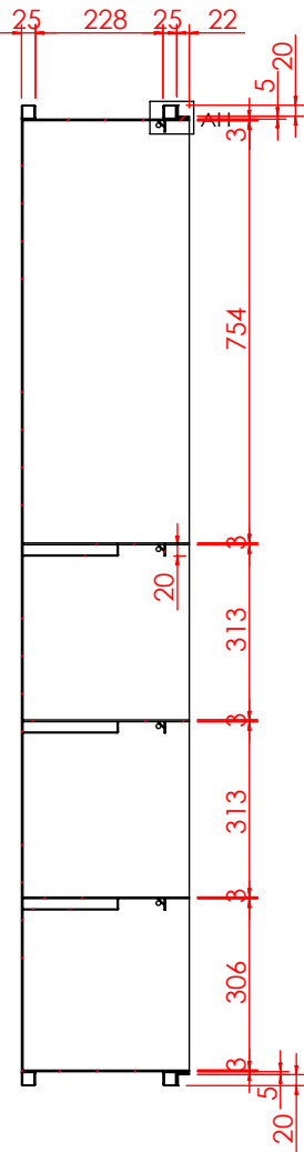
剖面 AG-AG
