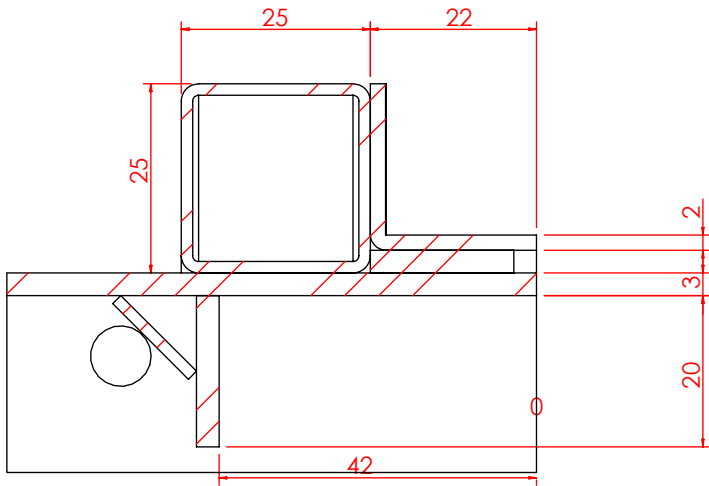
局部视图 AH 比例 1 : 1
