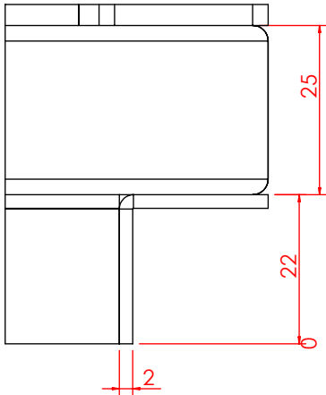
局部视图 AI 比例 1 : 1
