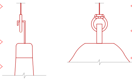
6 1:1 DETAIL
