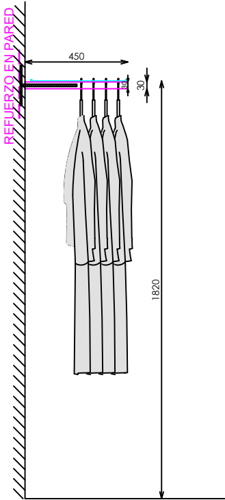
SECCION
