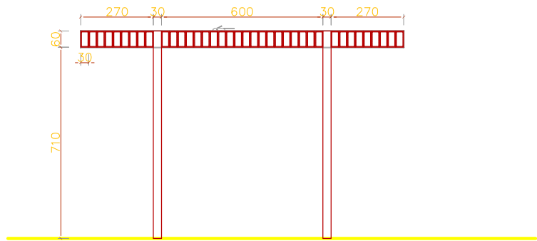
2 侧立面 1:10 PROFILE ELEVATION
