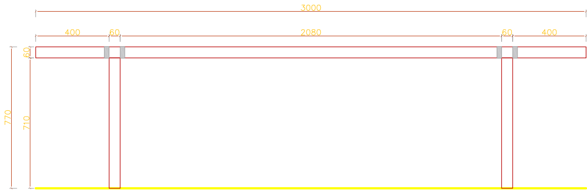
1 正立面 1:10 FRONT ELEVATION
