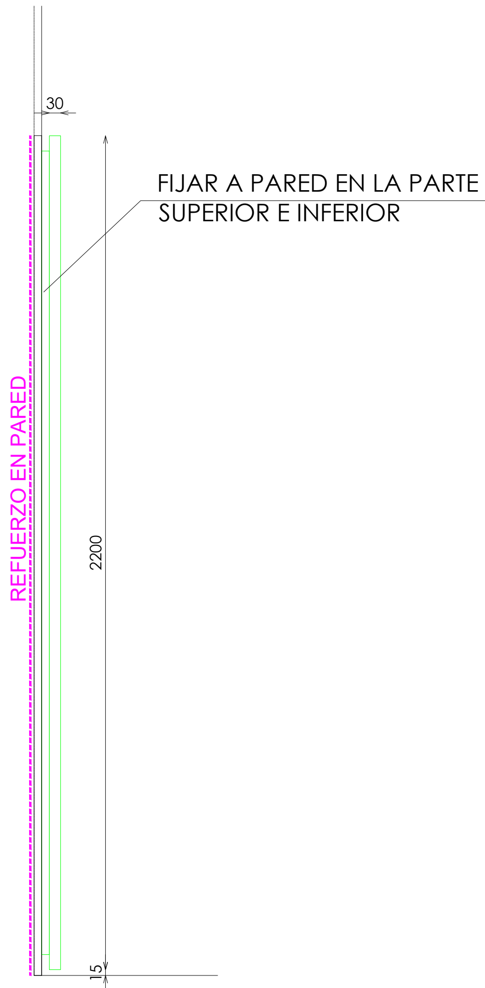
PERFIL
