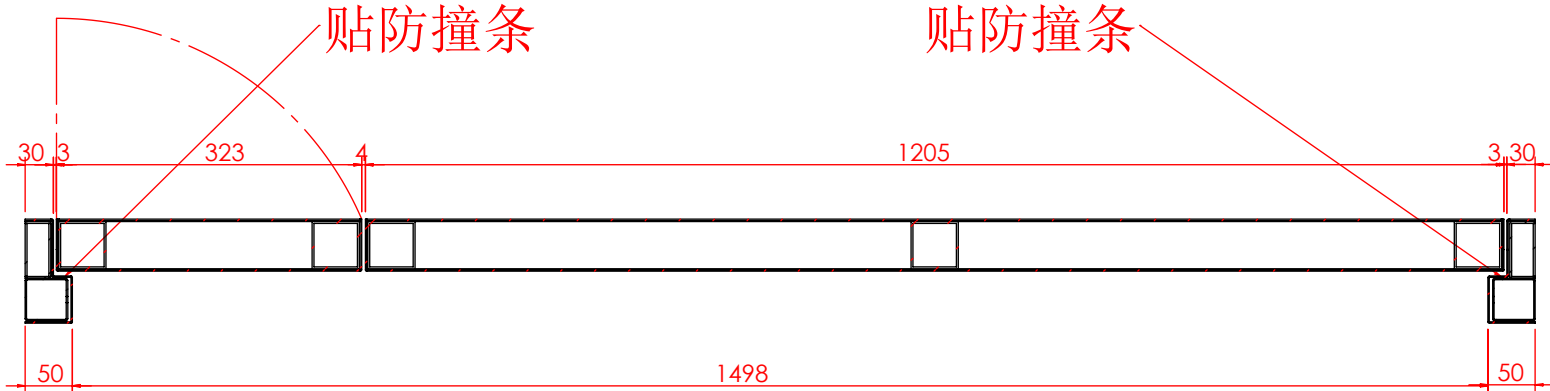
剖面 AH-AH 比例 1:8
