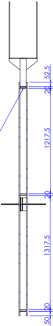
剖面 AG-AG
