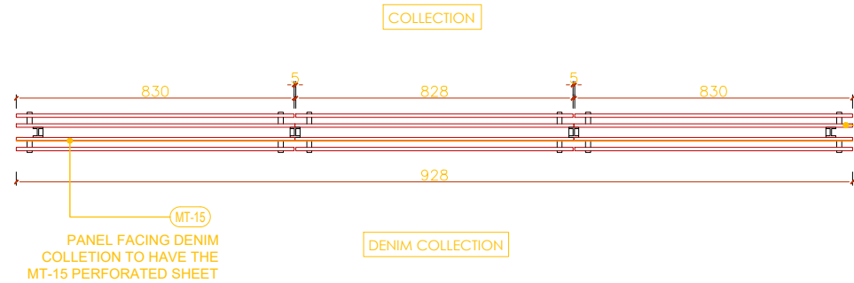
1 正立面 1:10 FRONT ELEVATION
