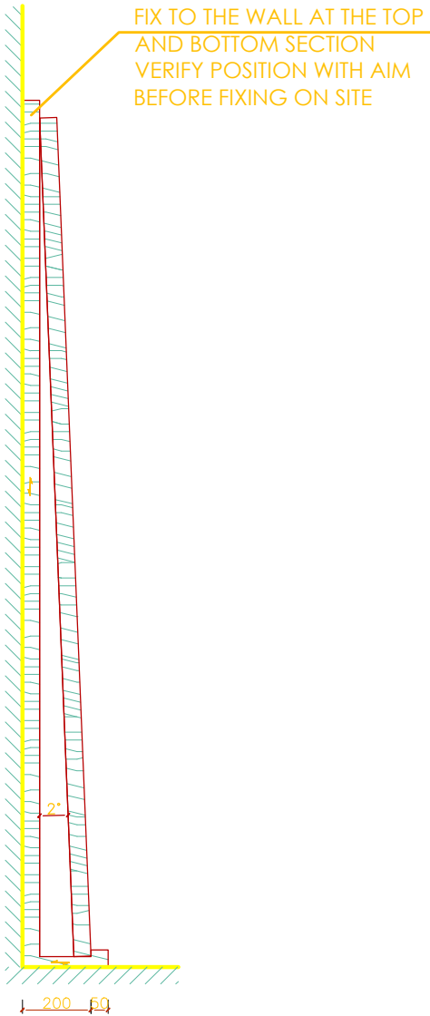
3 侧立面 1:10 SIDE ELEVATION
