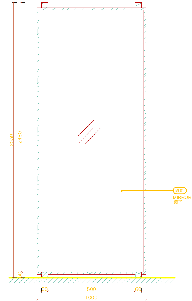
2 正立面 1:10 FRONT ELEVATION
