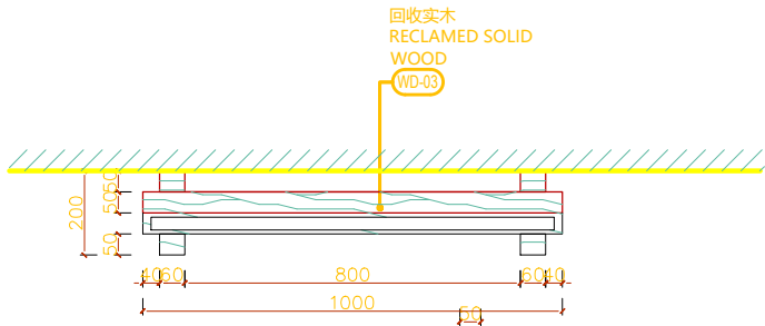
1 平面图 1:10 PLAN
