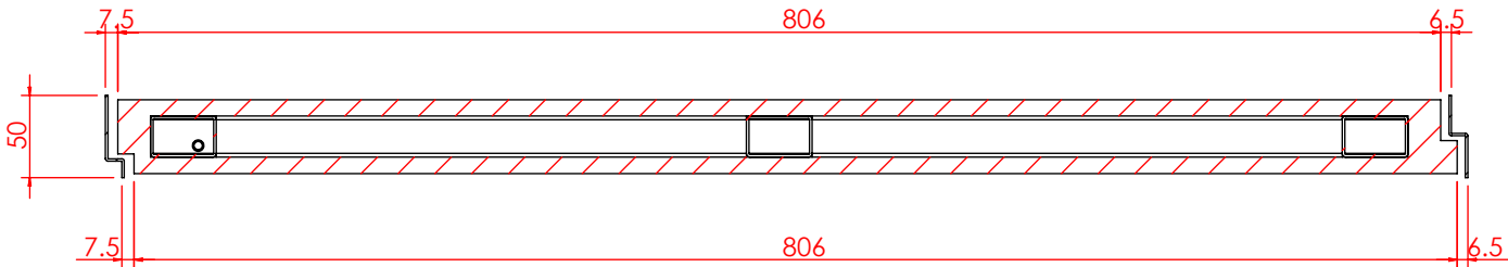
剖面 AH-AH 比例 1 : 5
