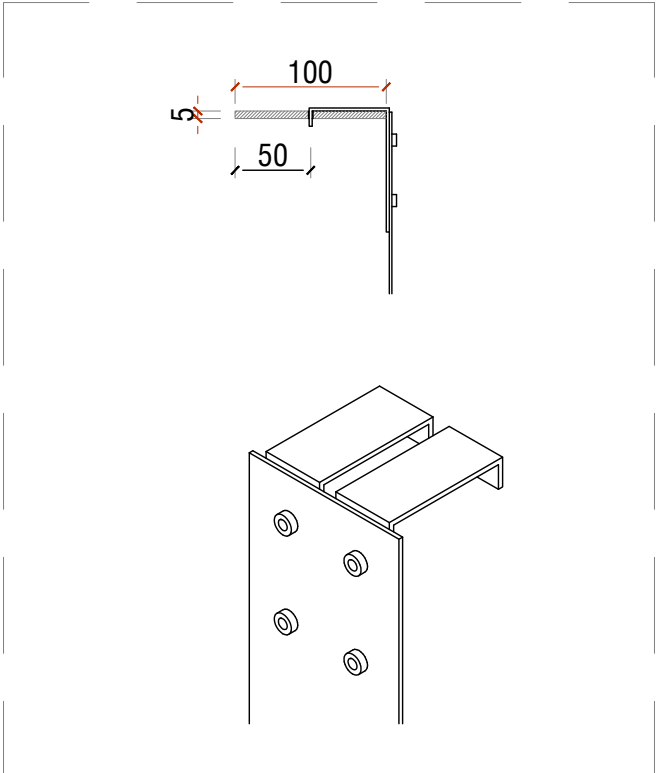
DETALLE ANCLAJE
