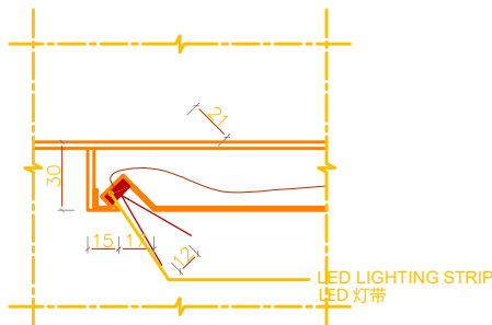
4 节点 1:2 DETAIL
