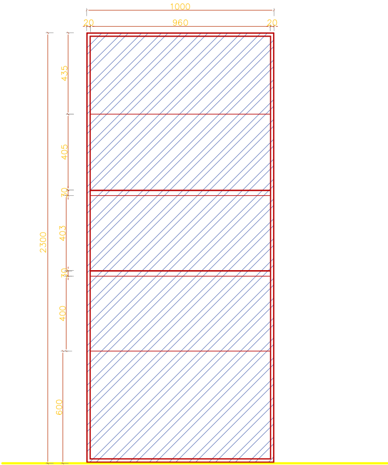
2 正立面 1:10 FRONT ELEVATION
