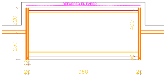
1 平面图 1:10 PLAN
