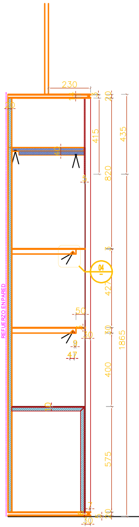
3 剖面图 1:10 SECTION
