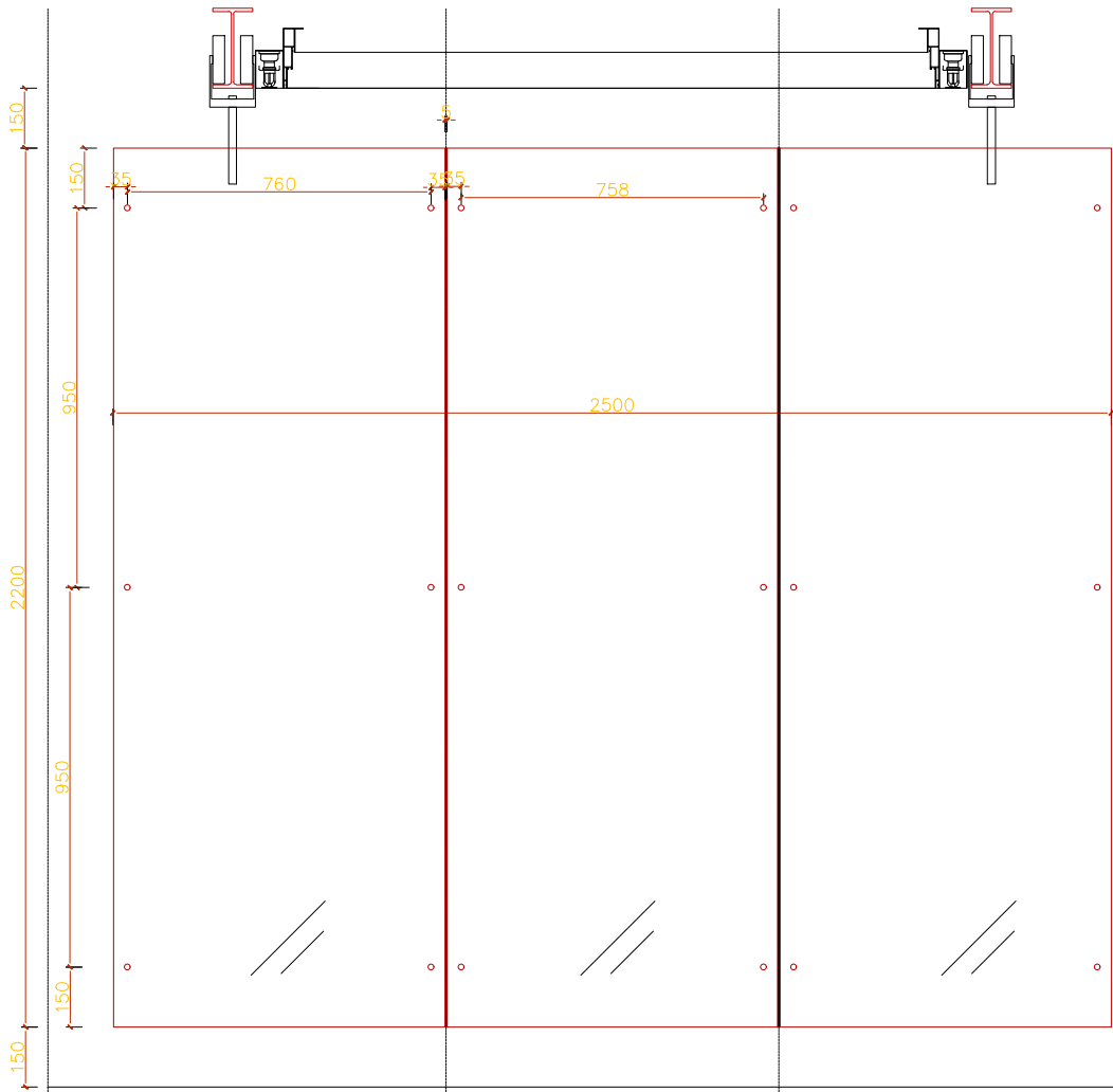
1 正立面 1:10 FRONT ELEVATION
