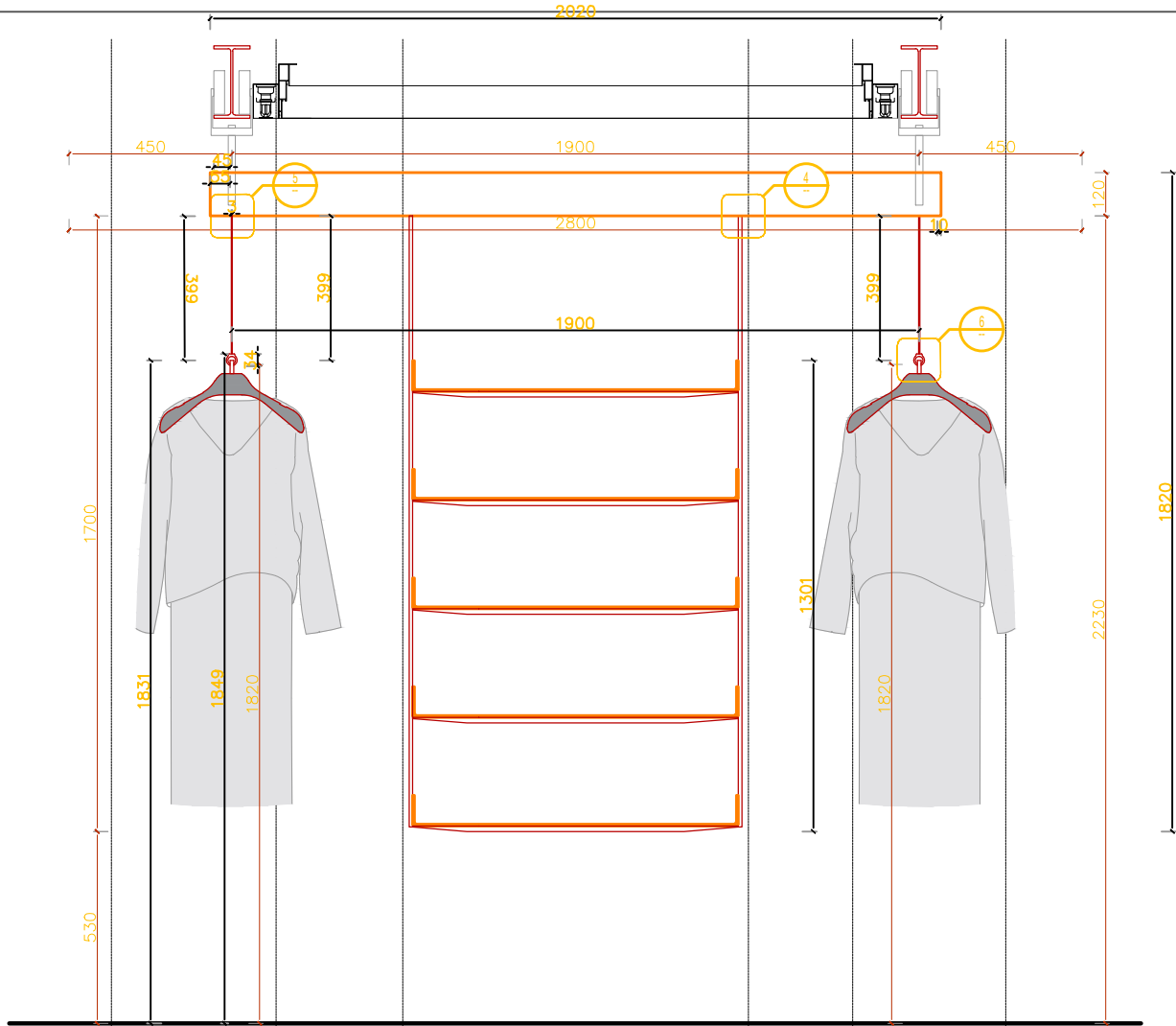
1 1:10 正立面 FRONT ELEVATION
