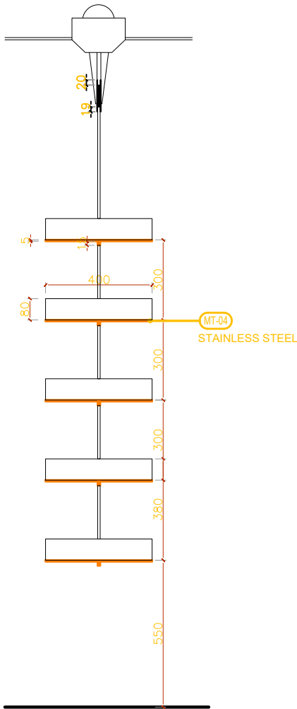
2 1:10 侧立面 SECTION
