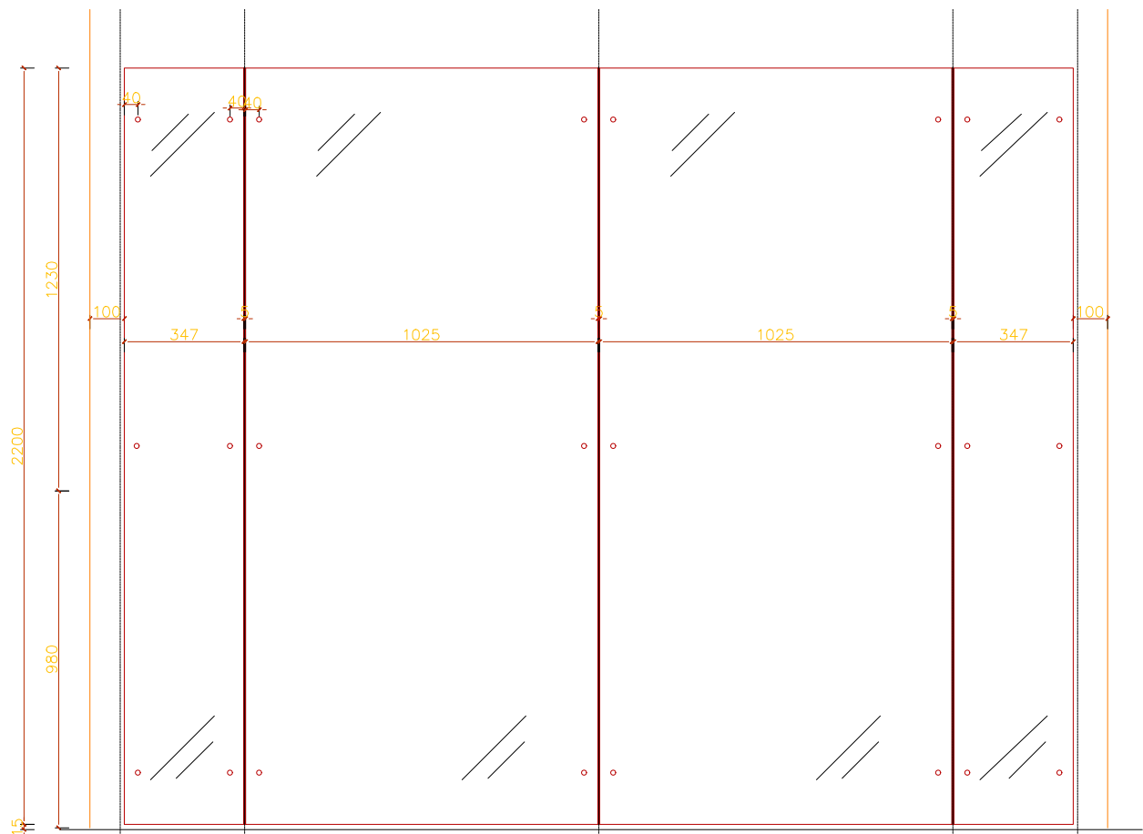
1 正立面 1:10 FRONT ELEVATION
