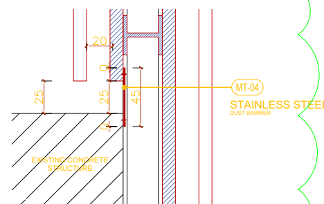
3 侧立面 1:2 JUNCTION DETAIL
