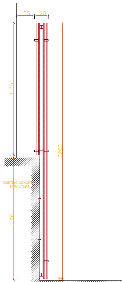
2 侧立面 1:10 SECTION
