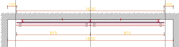
5 平面图 1:10 PLAN
