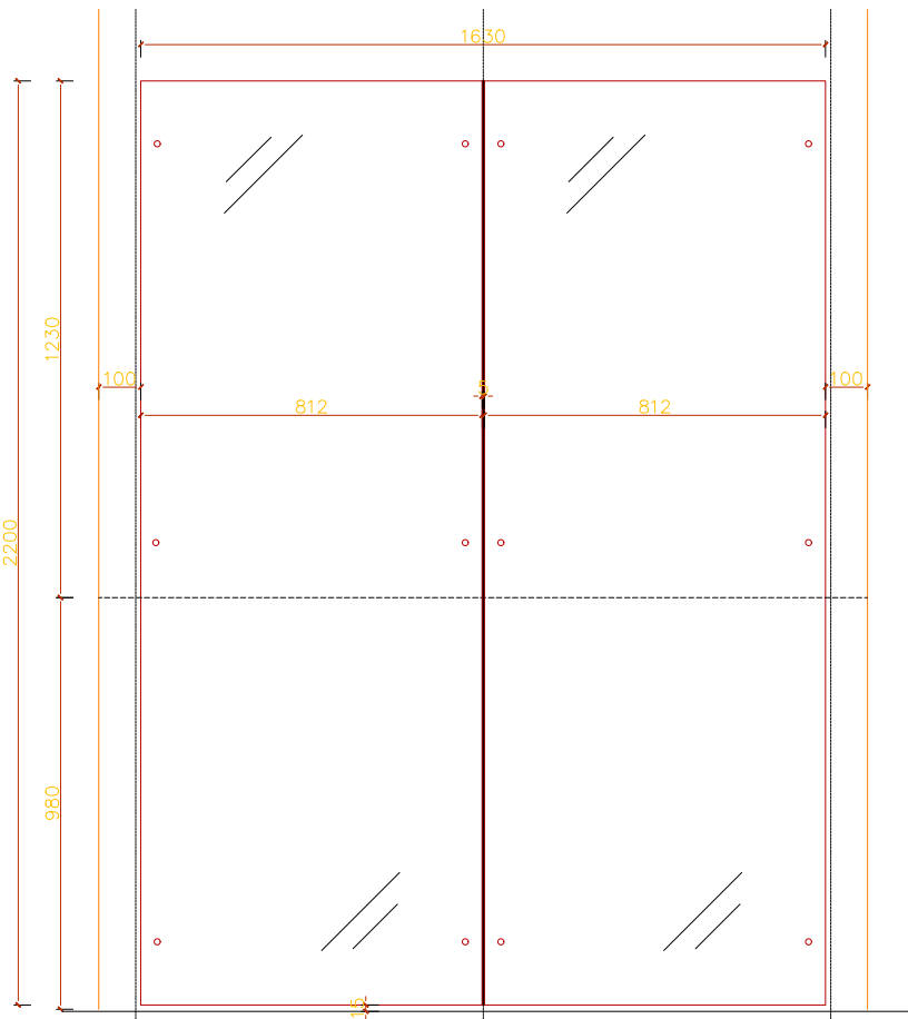
1 正立面 1:10 FRONT ELEVATION
