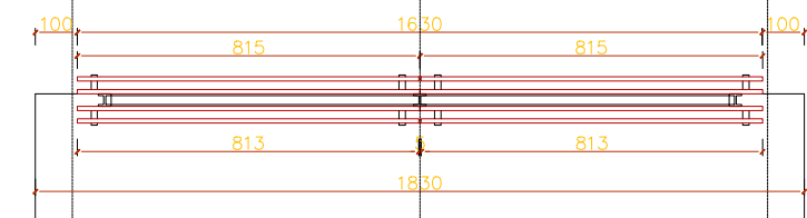
5 平面图 1:10 PLAN
