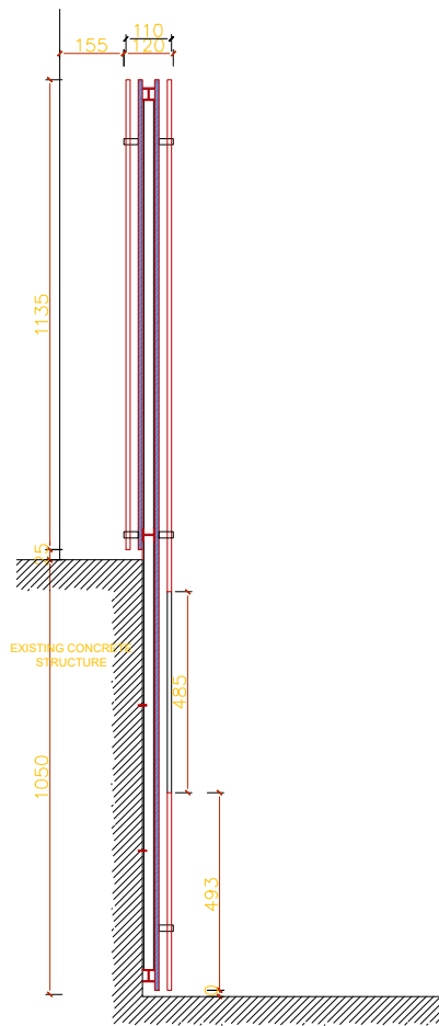
2 侧立面 1:10 SECTION
