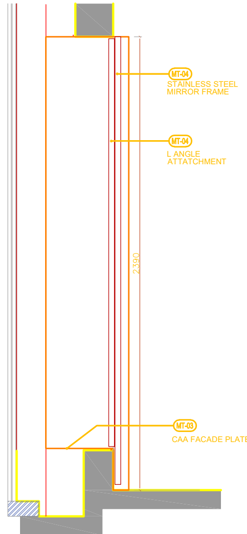
2 侧立面 1:10 SECTION
