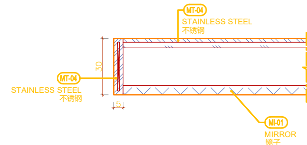
3 节点 1:1 DETAIL
