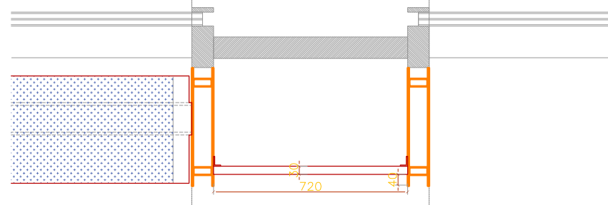
4 平面图 1:10 PLAN
