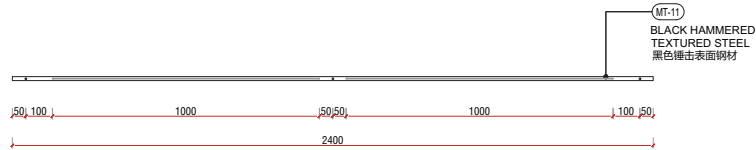
1 平面图 1:10 PLAN
