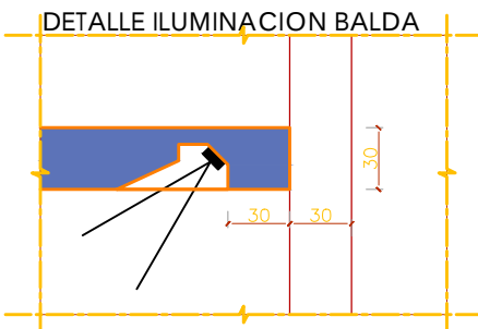
4 1:2 DETAIL
