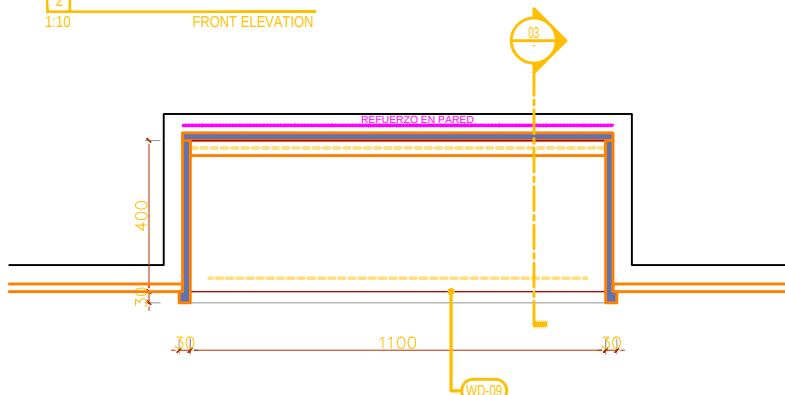
1 1:10 PLAN
