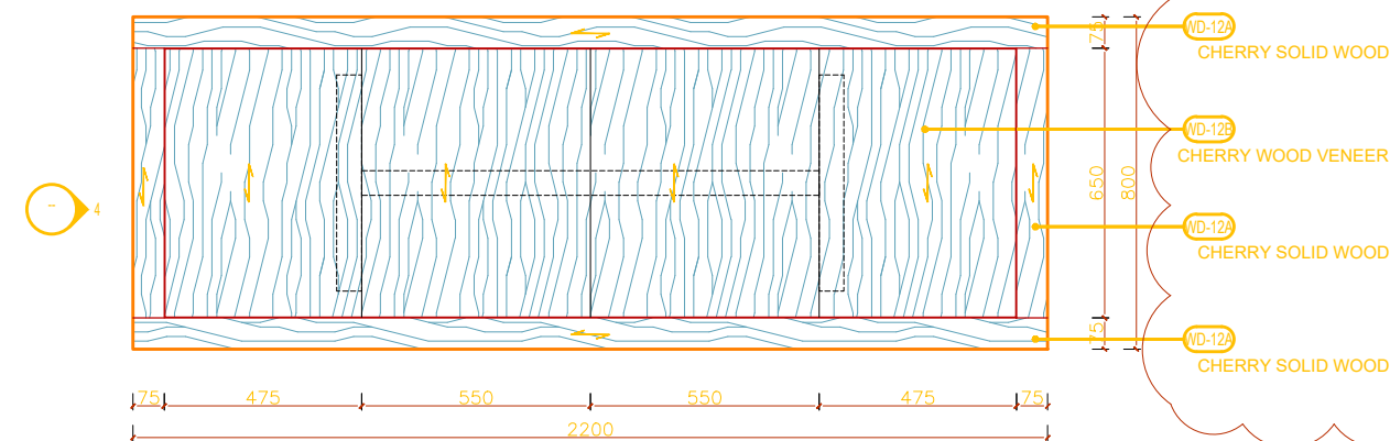
1 平面图 1:10 PLAN
