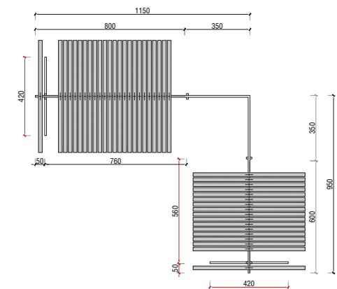
3 平面图 1:10 PLAN
