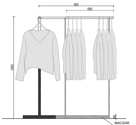
2 正立面 1:10 SIDE ELEVATION
