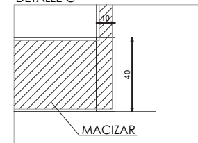
DETALLE C
