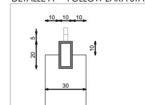
DETALLE B
