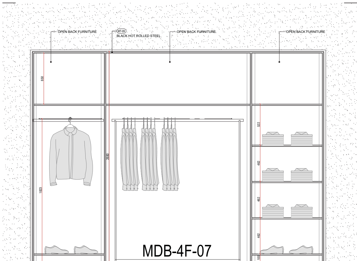
2 正立面 1:10 FRONT ELEVATION
