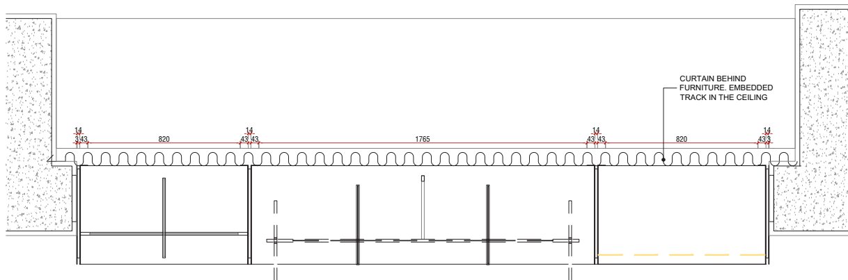
1 平面图 1:10 PLAN
