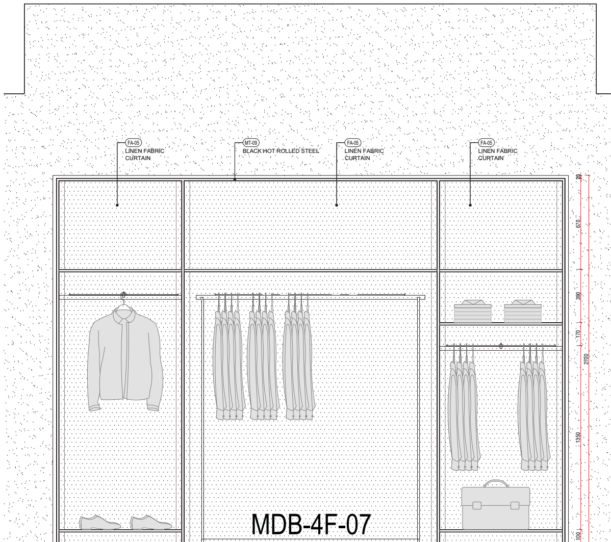
2 1:10 正立面 FRONT ELEVATION
