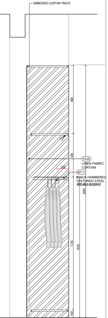
4 1:10 断面图 SECTION
