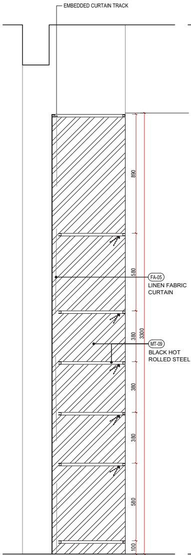
3 1:10 断面图 SECTION
