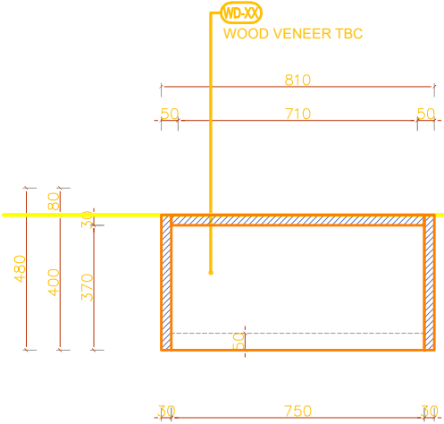
1 平面图 1:10 PLAN
