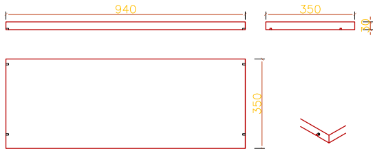
6 侧立面 1:10 DETAIL
