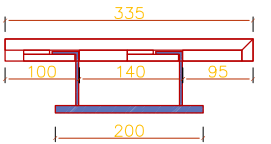
5 侧立面 1:10 DETAIL
