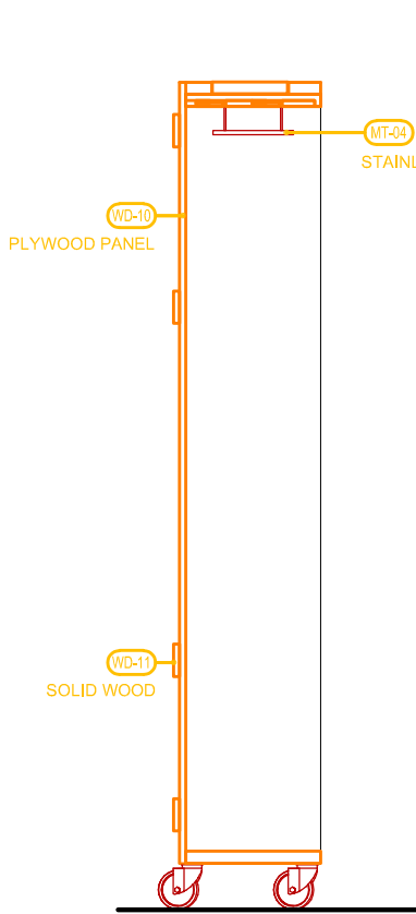
4 侧立面 1:10 LEFT BOX SECTION
