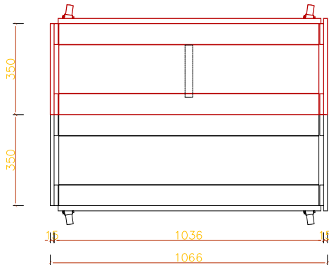
7 平面图 1:10 PLAN
