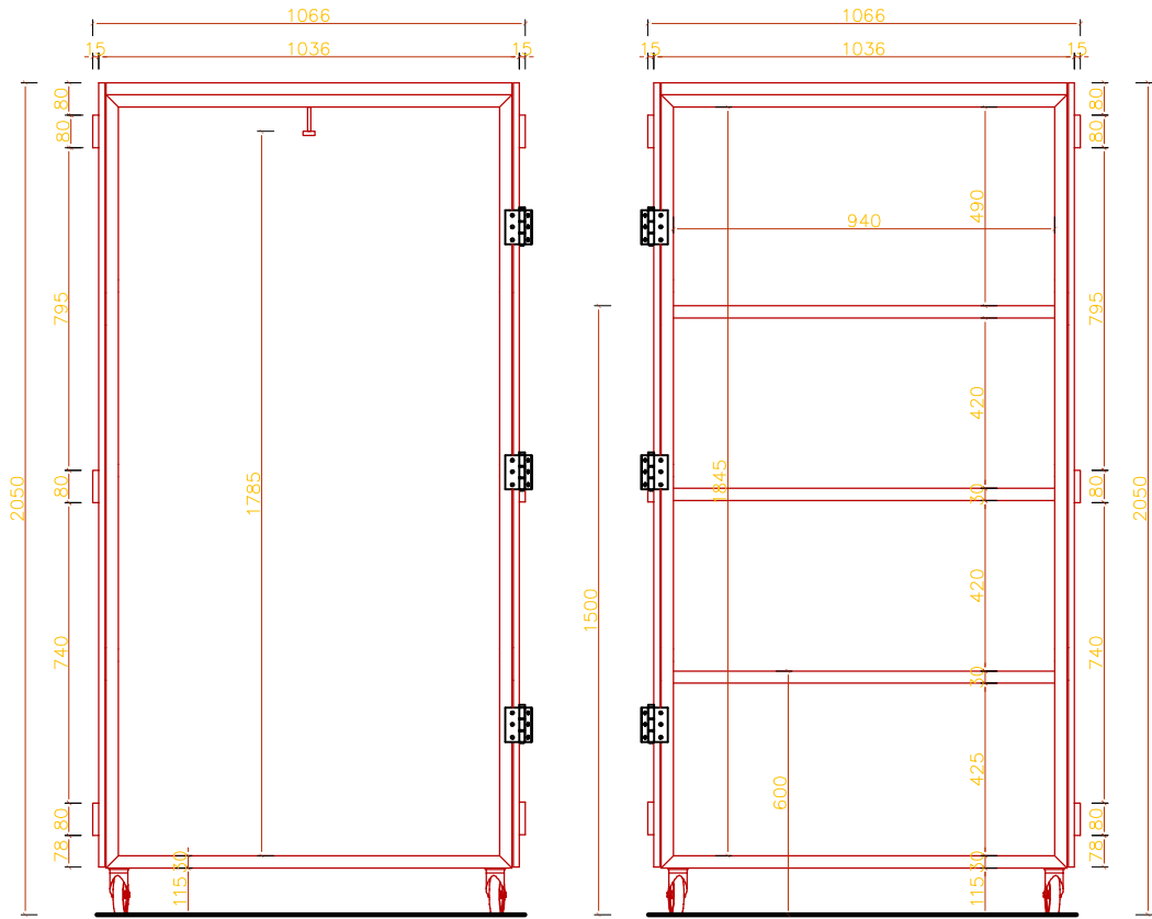
1 正立面 1:10 LEFT BOX FRONT ELEVATION
