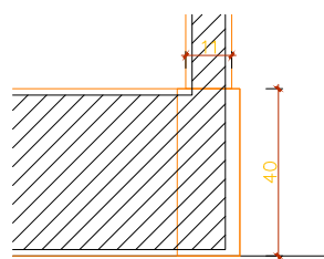
5 1:1 侧立面 DETAIL SOLID SUPPORT
