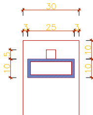
4 1:1 侧立面 DETAIL BAR
