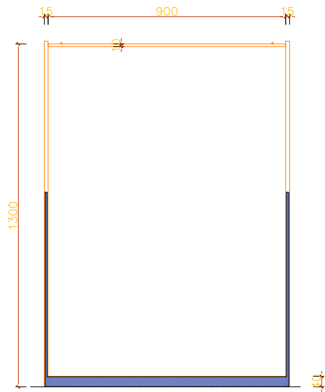
2 1:10 正立面 FRONT ELEVATION
