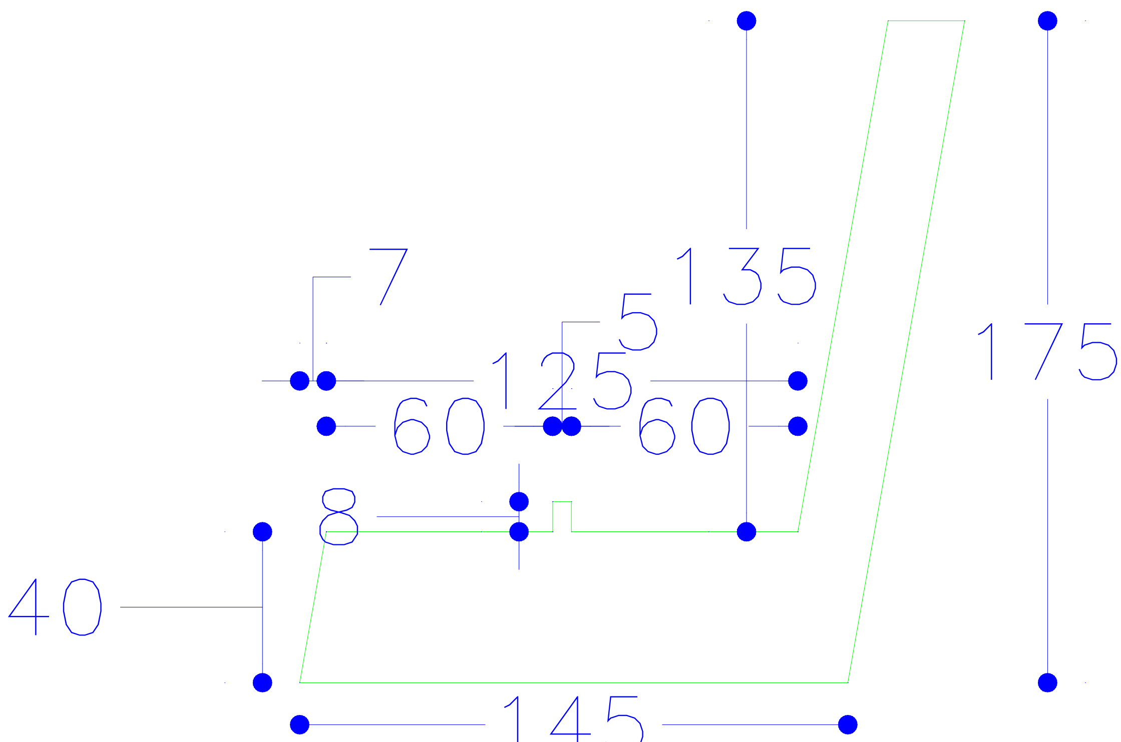
ALZADO
