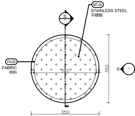
1 平面图 1:5 PLAN
