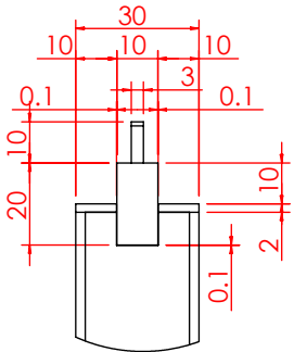
局部视图 AG 比例 1 : 2
