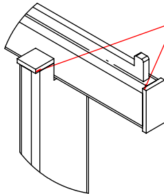
局部视图 AP 比例 1 : 2
