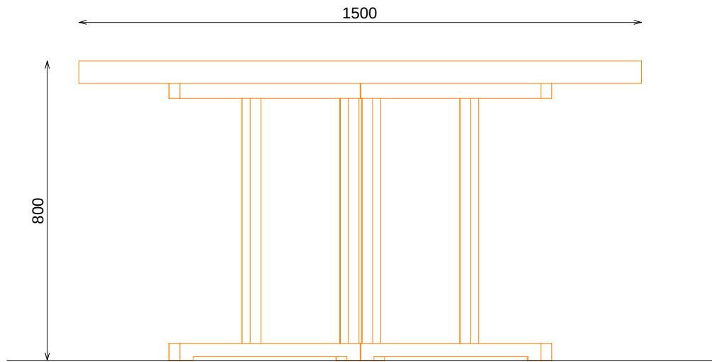
ALZADO FRONTAL
