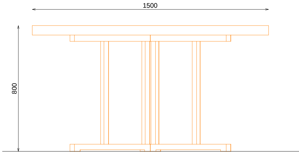
ALZADO LATERAL
