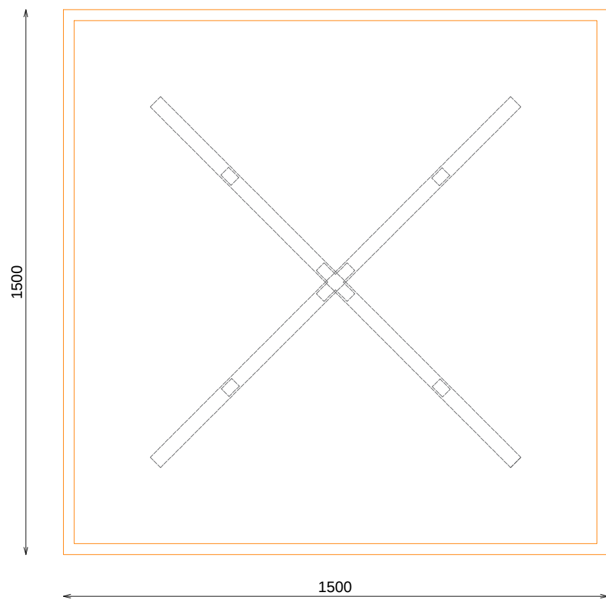
PLANTA
