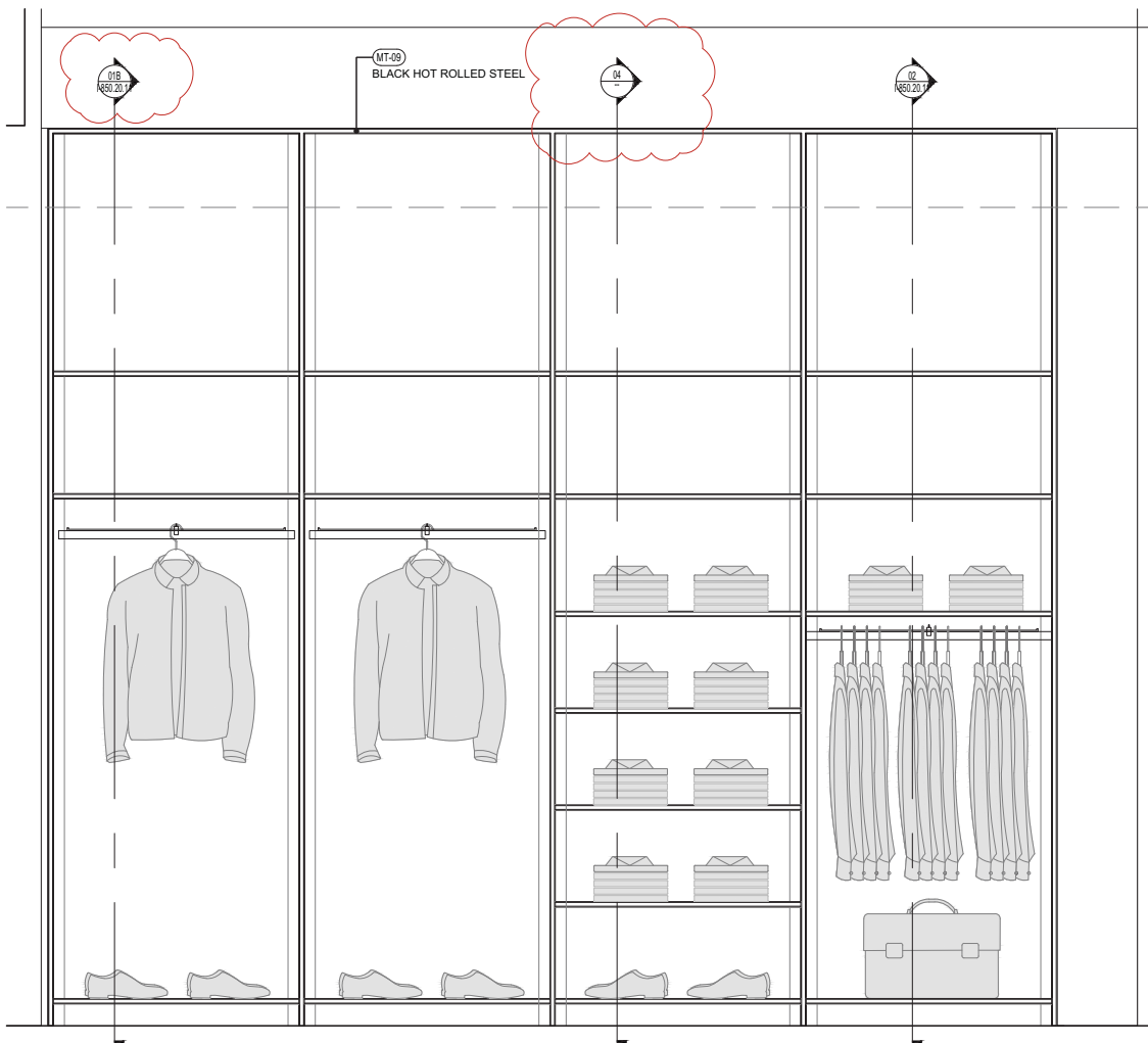
2 1:10 正立面 FRONT ELEVATION
