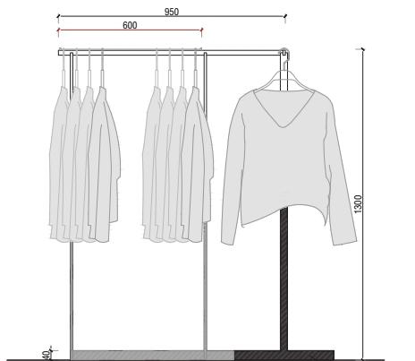
2 正立面 1:10 SIDE ELEVATION
