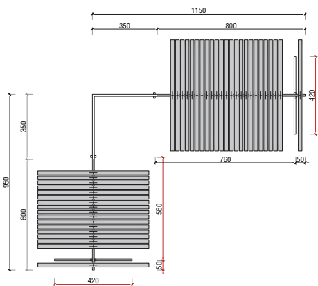
3 平面图 1:10 PLAN
