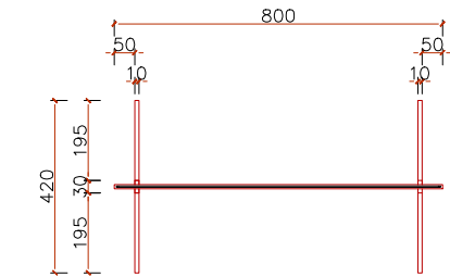
3 平面图 1:10 PLAN
