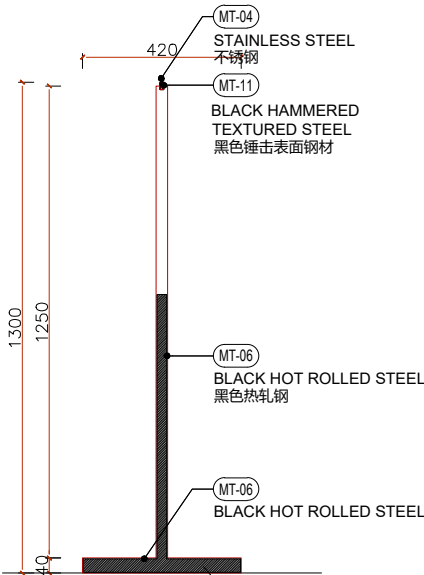
3 剖面图 1:10 SECTION
