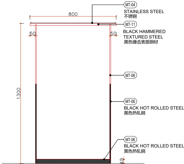
1 正立面 1:10 FRONT ELEVATION
