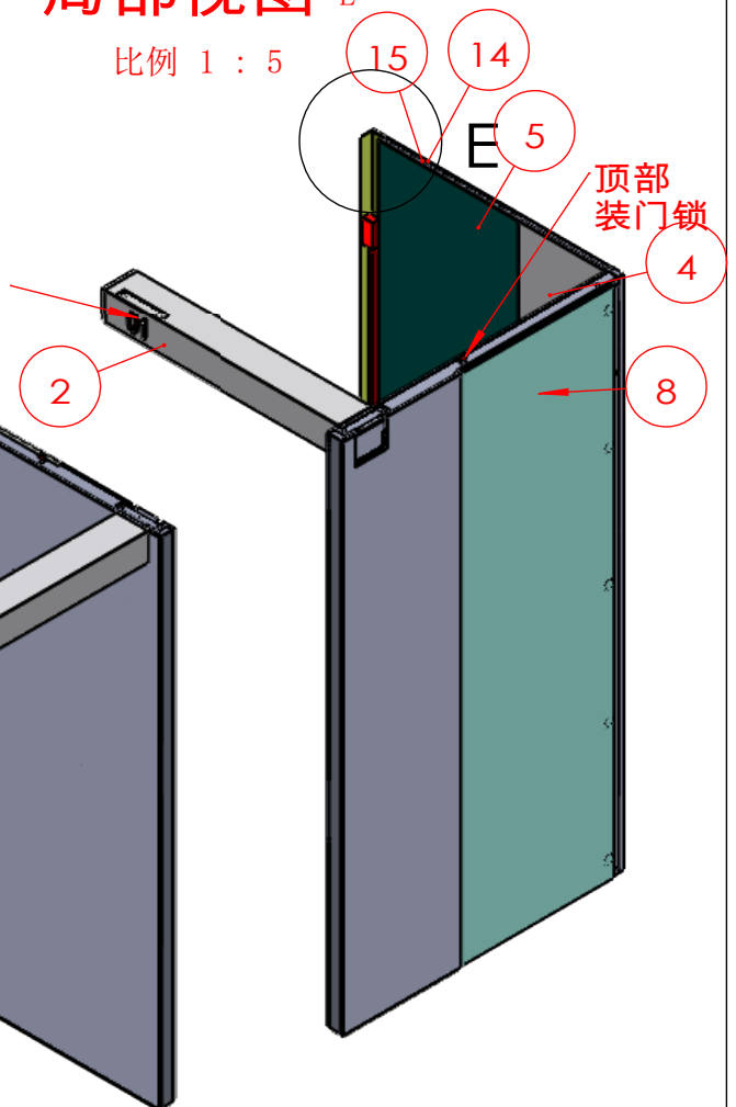
局部视图 E
