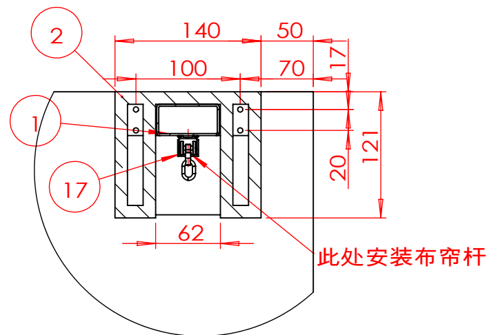
局部视图 D
