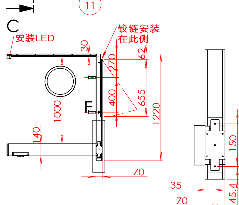
局部视图 F
