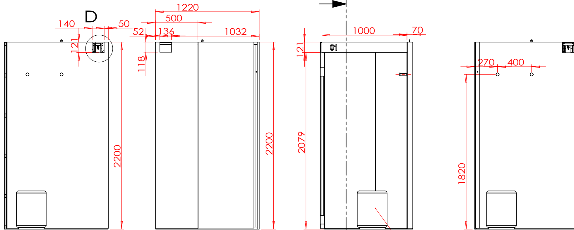
剖面 C-C
