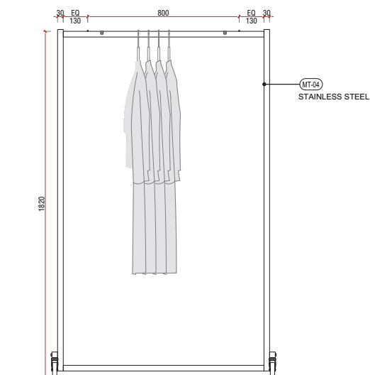
2 正立面 1:10 FRONT ELEVATION
