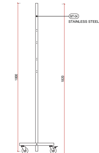
3 侧立面 1:10 PROFILE ELEVATION
