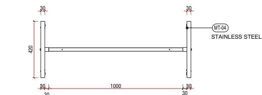
1 平面图 1:10 PLAN
