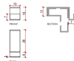
7 节点 1:1 DETAIL DOTACION FRONTAL
