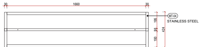
1 平面图 1:10 PLAN
