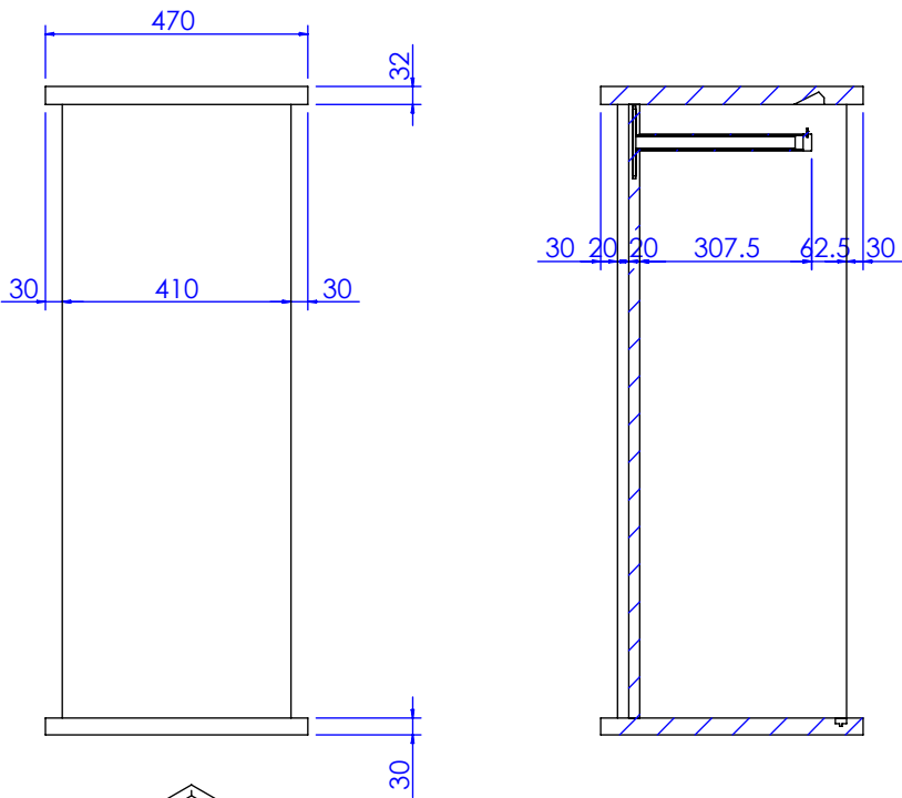
剖面 AG-AG
