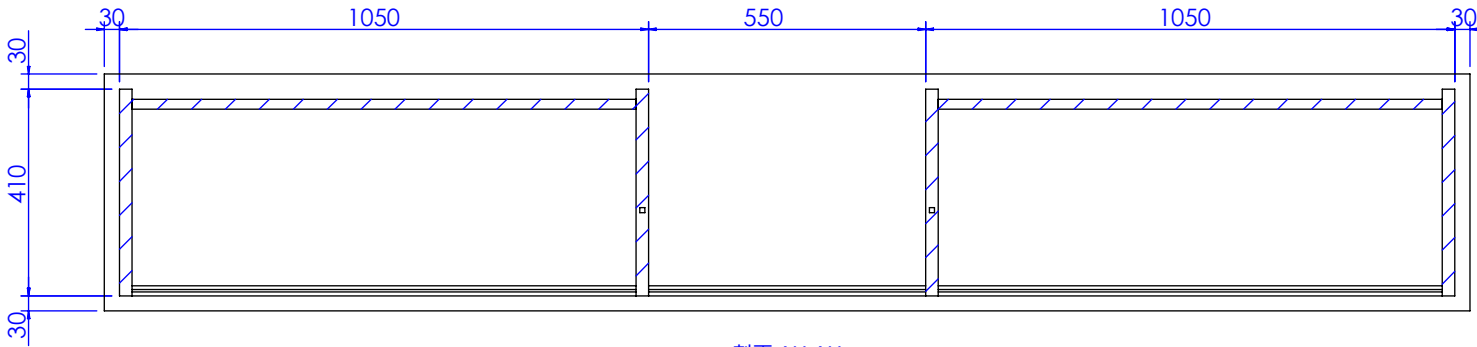
剖面 AH-AH
