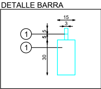
DETALLE BARRA
