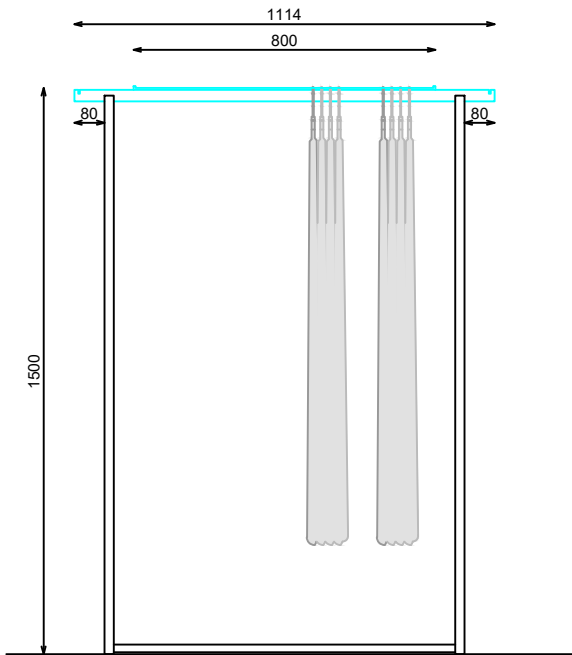
ALZADO
