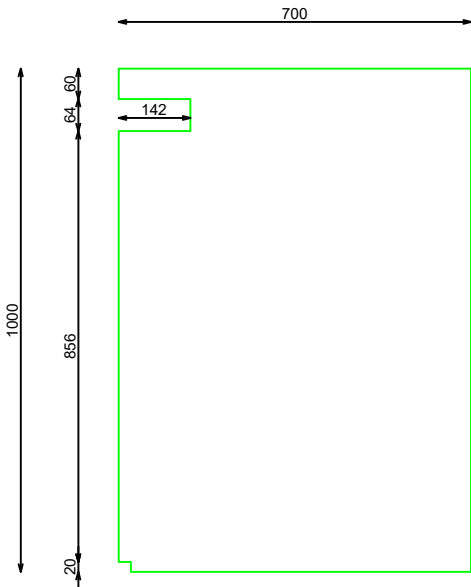
ALZADO B
