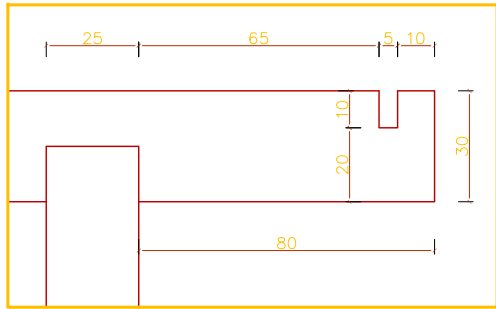
6 节点 1:2 DETAIL
