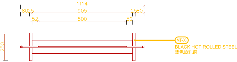
1 平面图 1:10 PLAN
