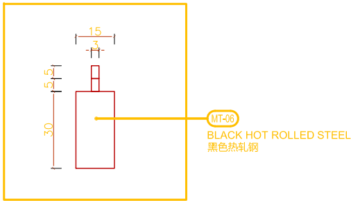
5 节点 1:2 DETAIL
