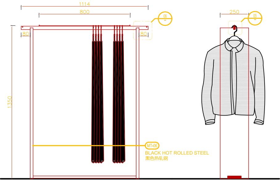
2 正立面 1:10 FRONT ELEVATION
