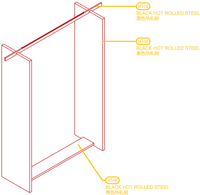
4 轴侧 AXON
