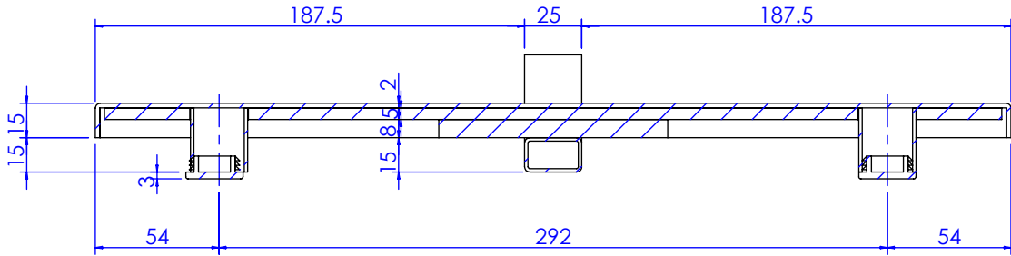
局部视图 B 比例 1 : 3
