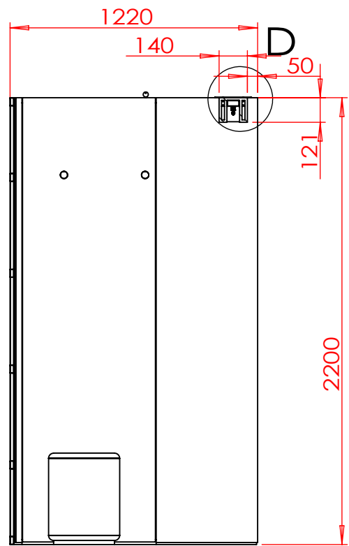
剖面 C-C
