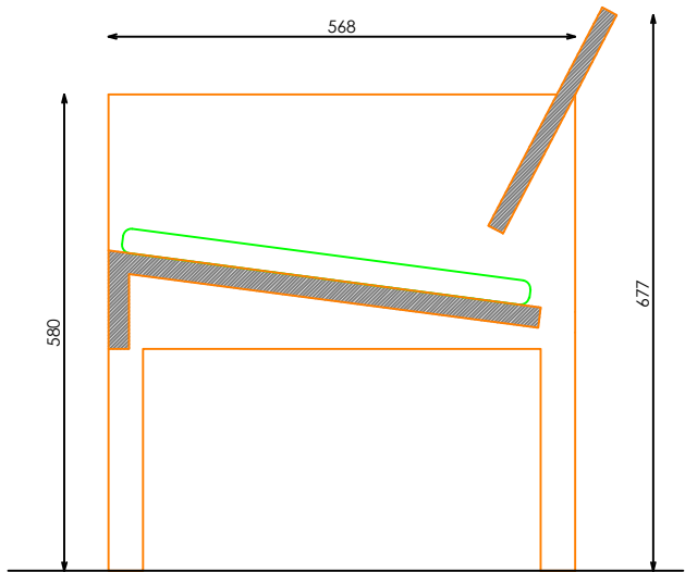
SECCIÓN
