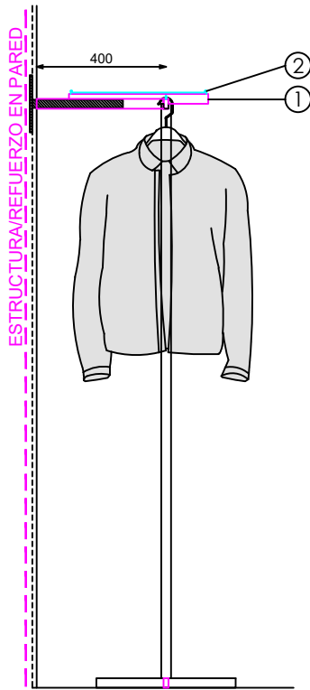
SECCION
