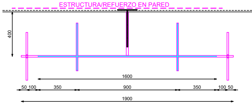
PLANTA
