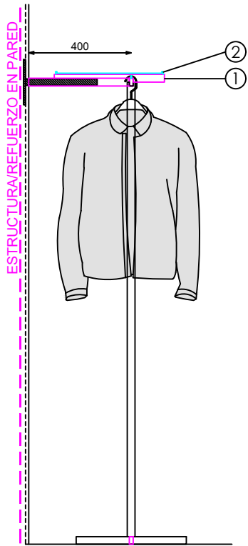
SECCION
