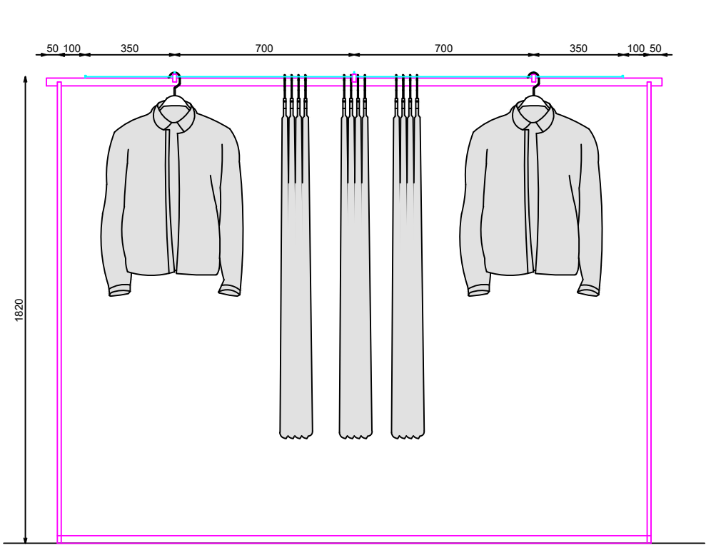
ALZADO
