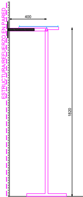
SECCION
