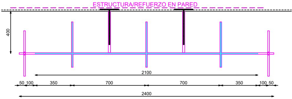
PLANTA
