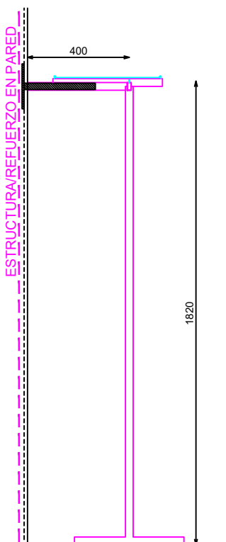
SECCION
