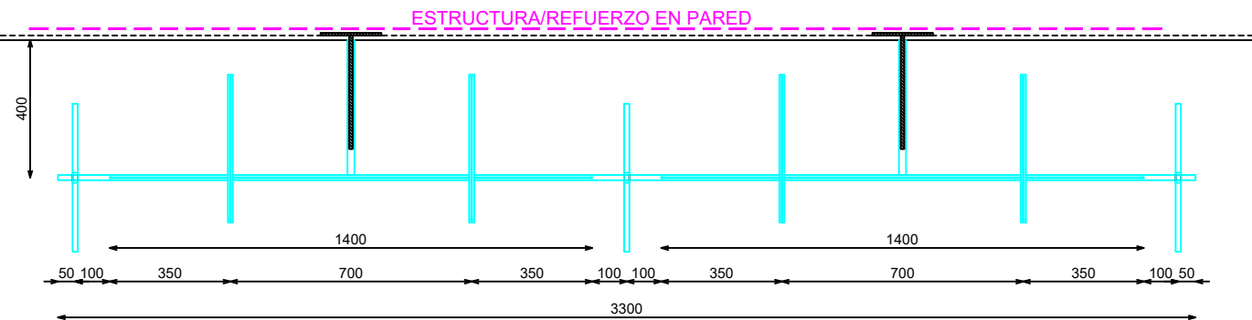
PLANTA
