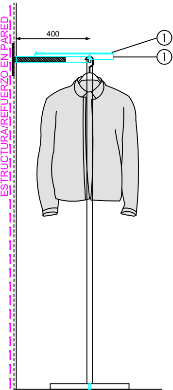
SECCION
