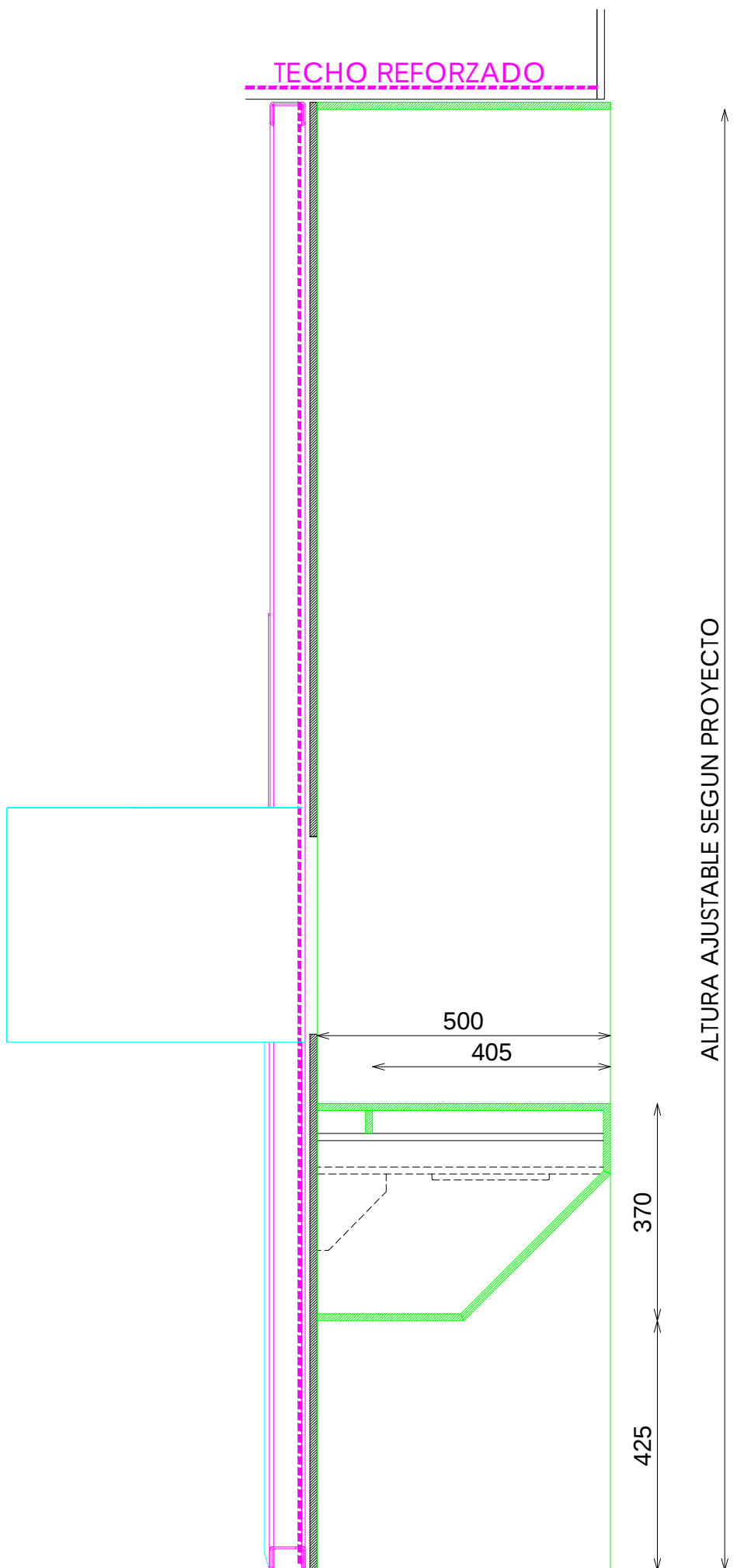
SECCIÓN
