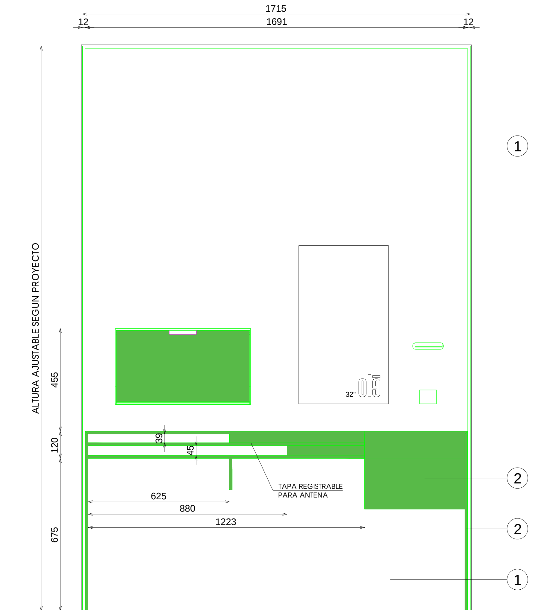
ALZADO FRONTAL
